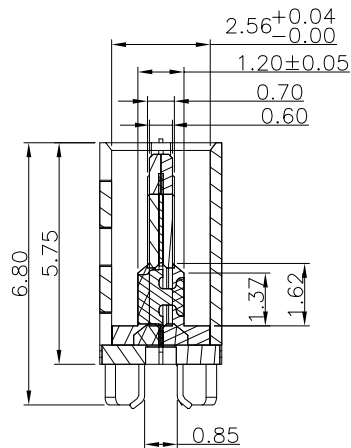
截面 A-A
