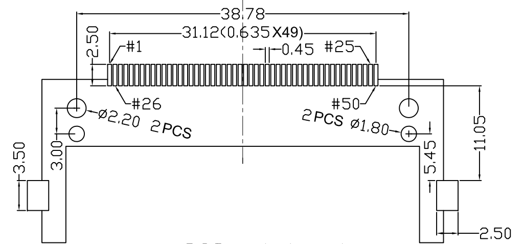
P.C.Board layout
