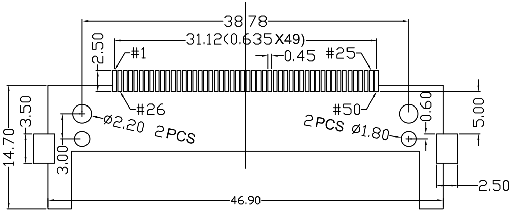
P.C.Board layout
